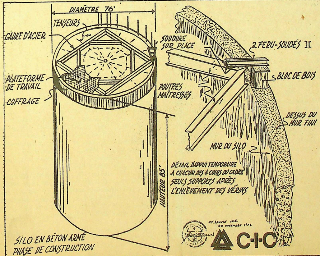
La rappresentazione ci-dessus réalisée par l'ingénieur du CIC, M. N. Y. Lavoie, indique que la tragédie du Mont Wright s'est déroulée lorsque la soudure reliant deux fers en "U" à la plate-forme de travail a cédé. On voit à gauche le silo qui
